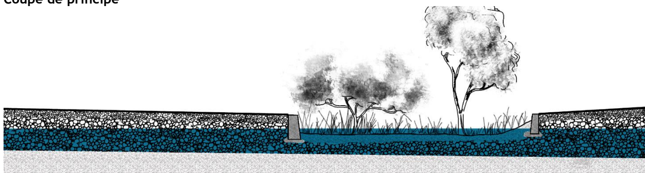
Massif d'infiltration unique entre une noue et une structure de voirie
