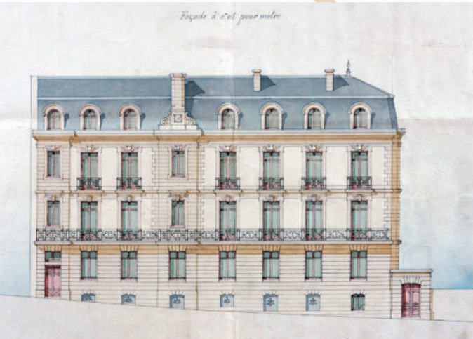
Développé des élévations sur rue de l'hôtel particulier Taslé, 6 place de la République, 24 rue Thiers (Vannes), 1888, par E. Bassac (?). Fonds privé. © Ville de Vannes
